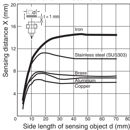
E2AU-M30 S15/ E2A-S30 S15
