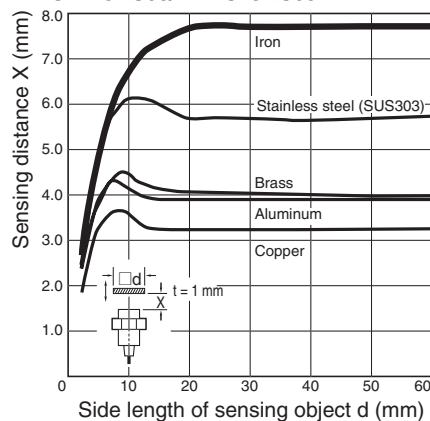
E2AU-M18 S08/E2A-S18 S08
